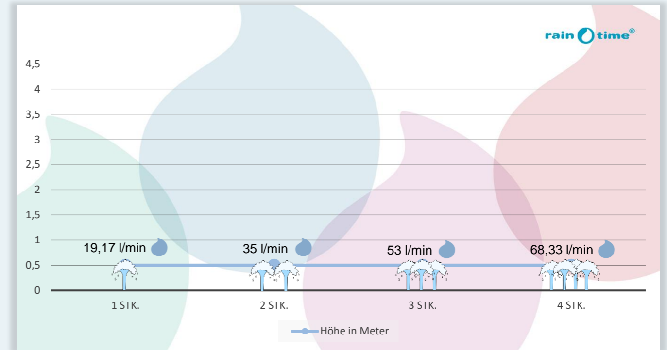
Verbrauch von 1 bis 4 Schaumdüse (l/min) bei einer Höhe von 0,5 Metern
