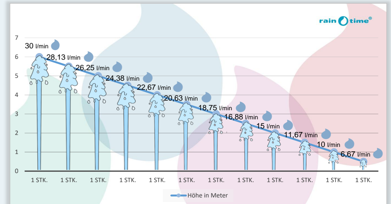
Verbrauch einer Strahldüse (l/min) in Abhängigkeit von der Höhe
