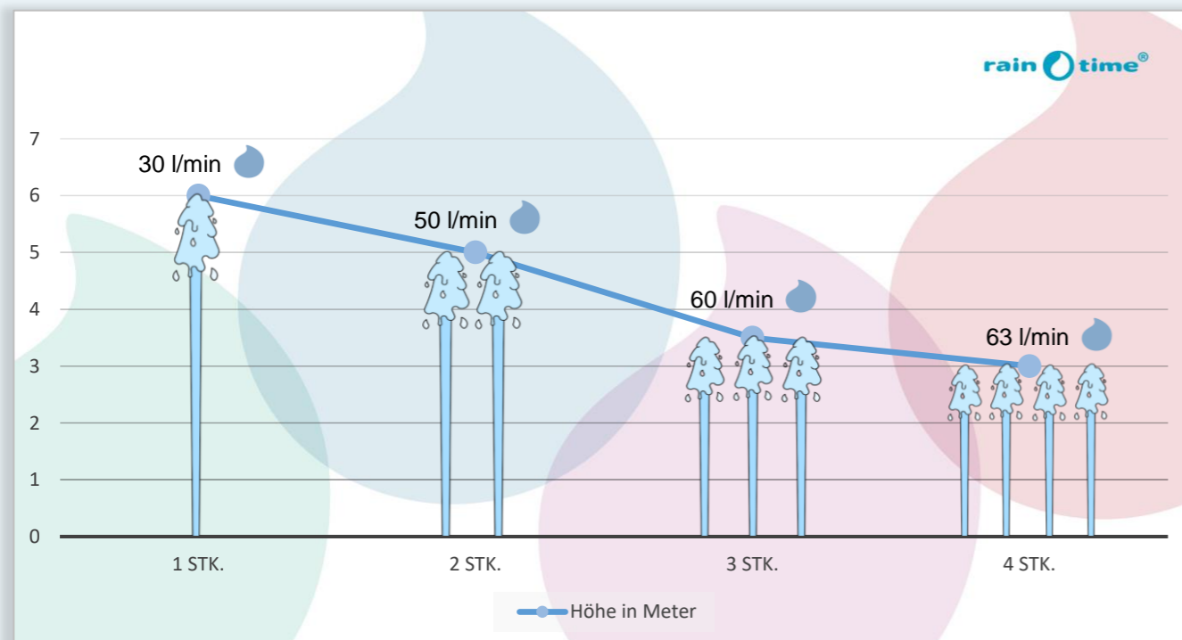
Verbrauch einer Strahldüse (l/min) bei vollständiger Auslastung der Pumpe mit maximal 4,2 bar, etwa 4200 Liter pro Stunde
