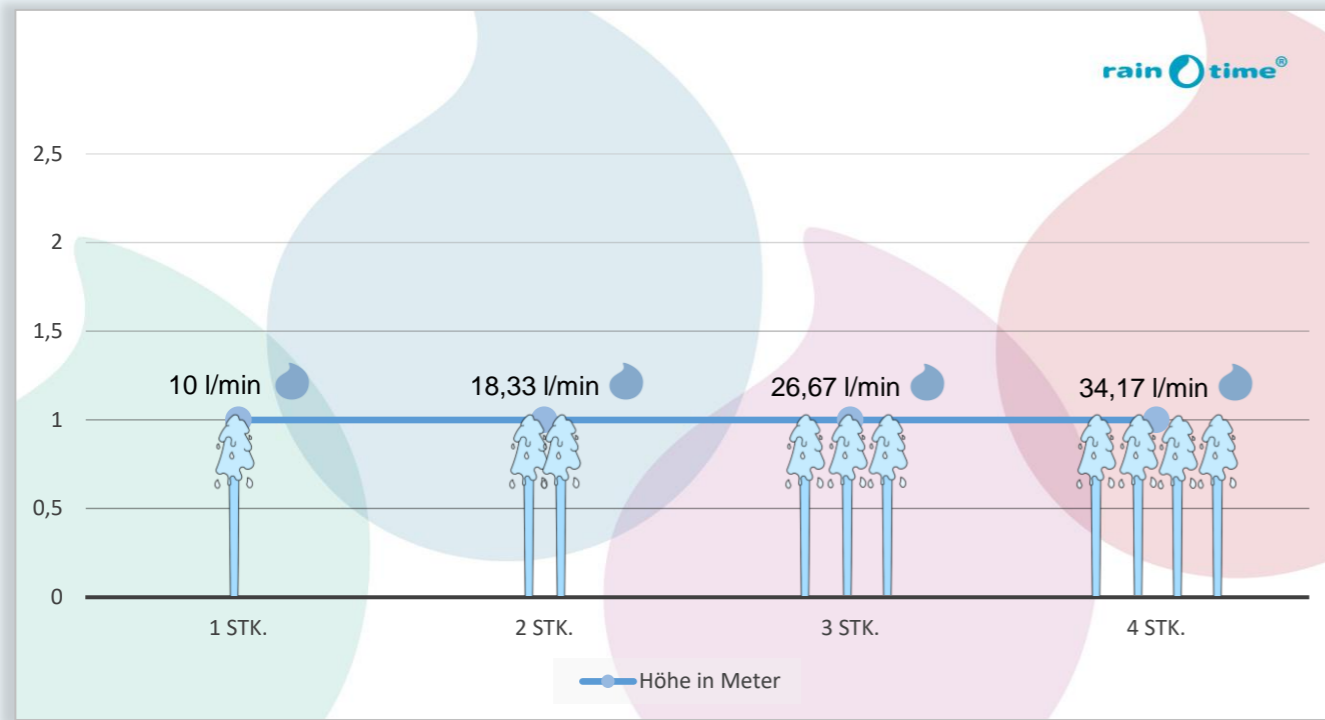
Verbrauch von 1 bis 4 Strahldüsen (l/min) bei einer Höhe von 1 Meter
