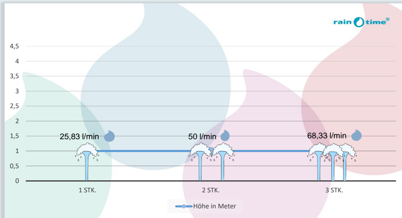
Verbrauch von 1 bis 4 Schaumdüsen (l/min) bei einer Höhe von 1 Meter
