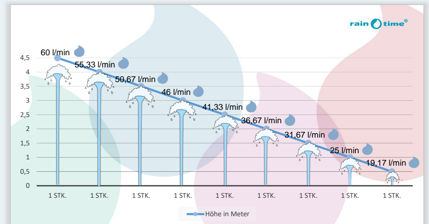
Verbrauch einer Schaumdüse (l/min) in Abhängigkeit von der Höhe
