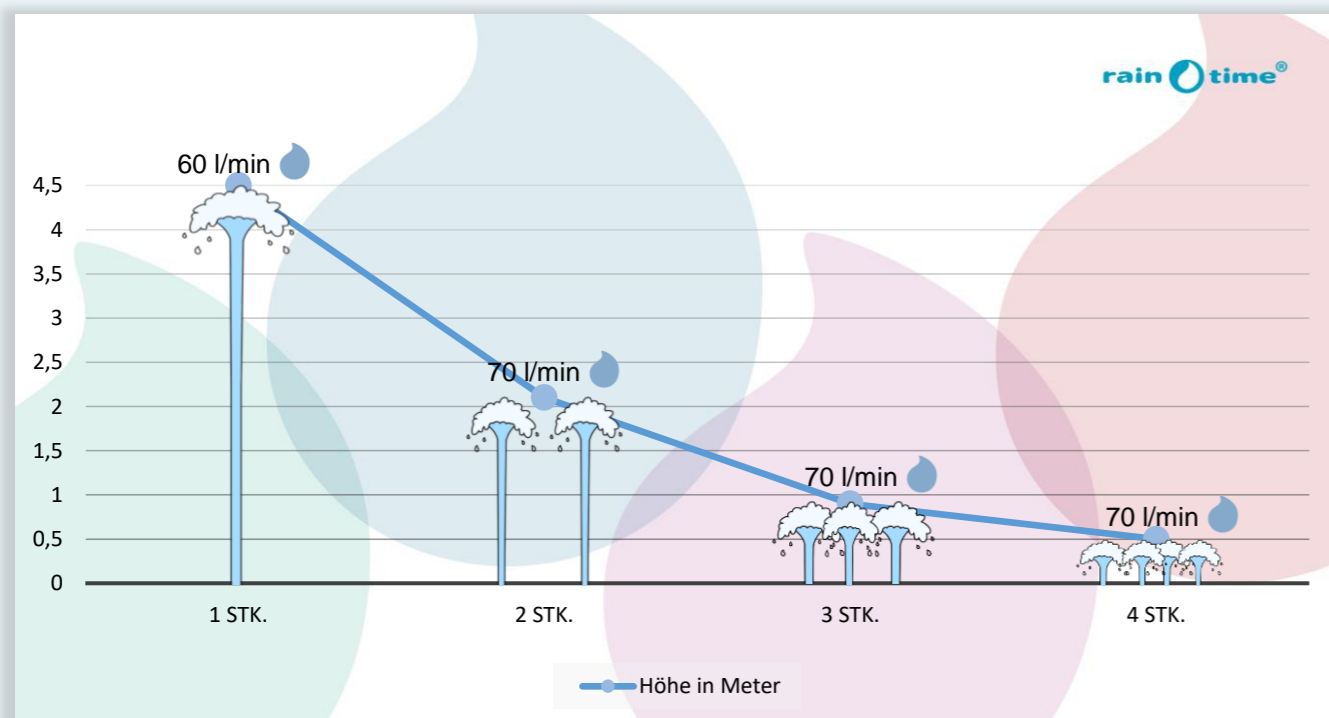
Verbrauch einer Schaumdüse bei vollständiger Auslastung der Pumpe mit maximal 4,2 bar, etwa 4200 Liter pro Stunde
